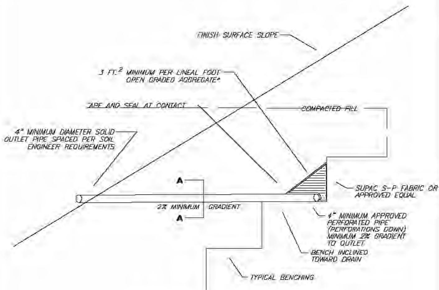
DETAIL A-A
