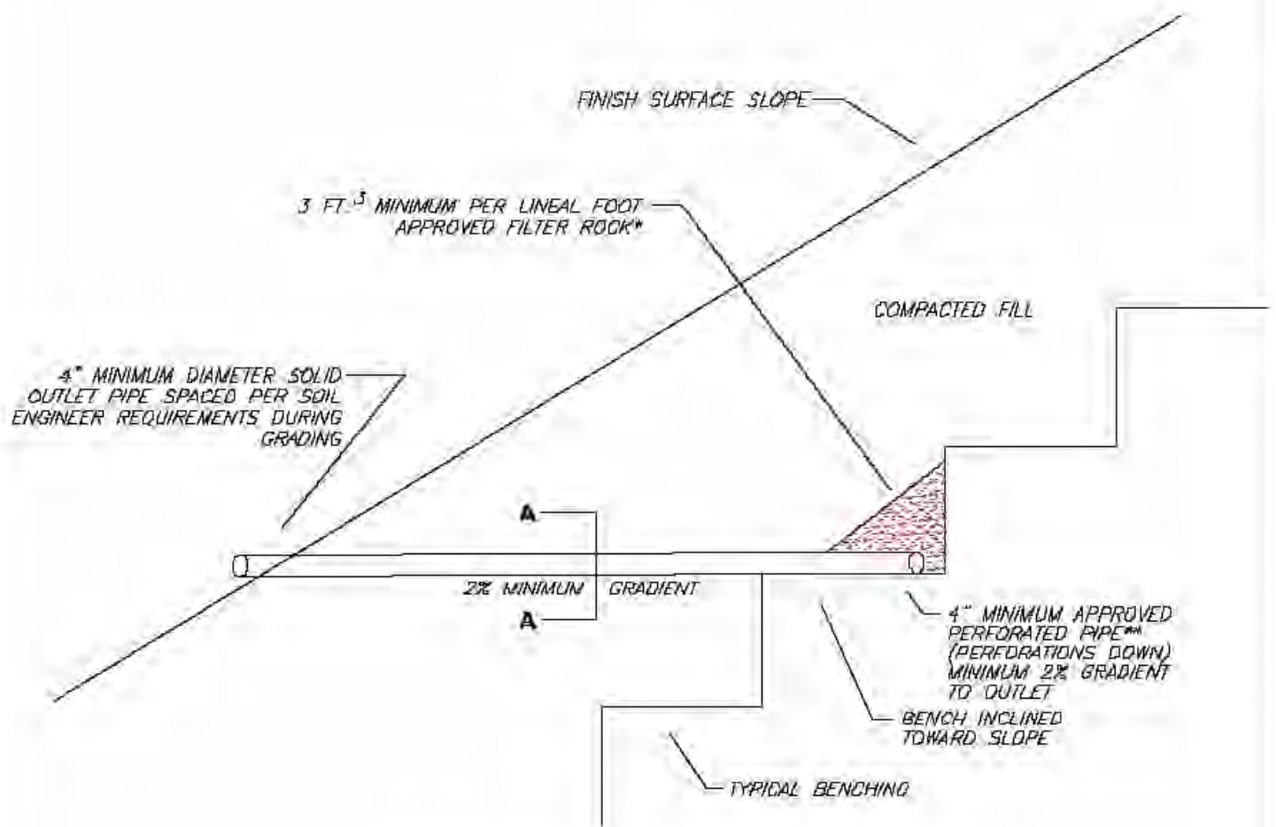
DETAIL A-A
